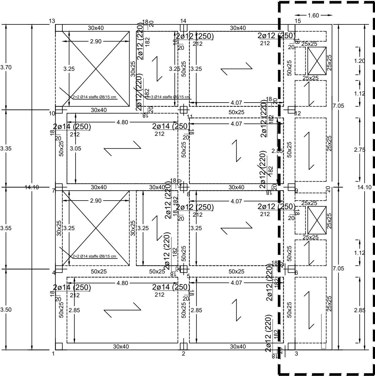
Pianta al livello 2 - Quota 6.95 m.
